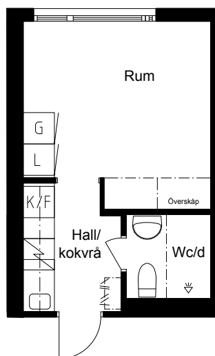
PLAN 1, Entréplan
