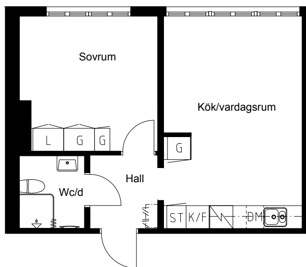
PLAN 1, Entréplan
